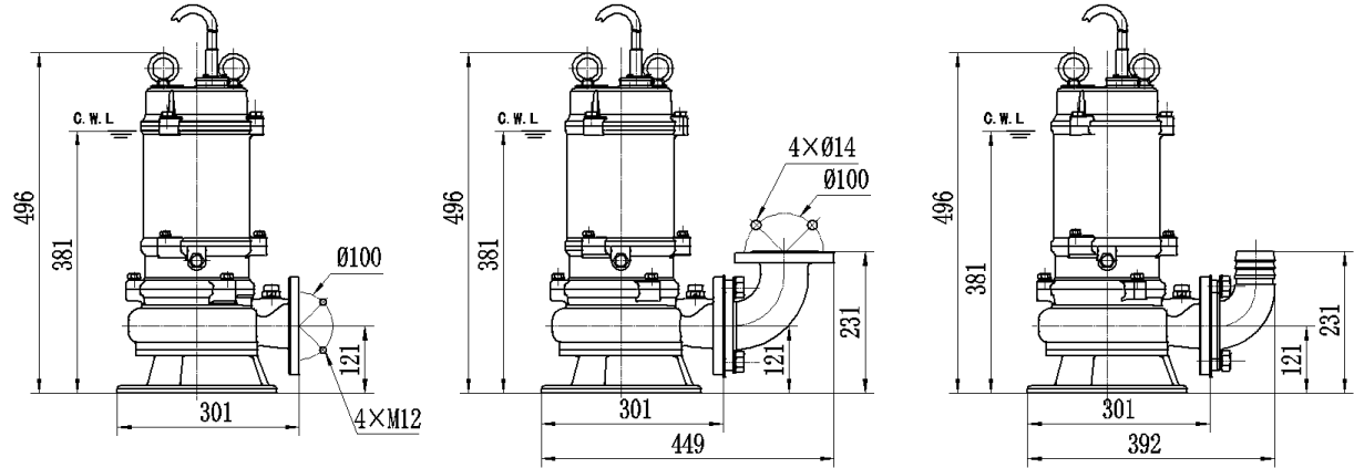
移动式安装尺寸图
