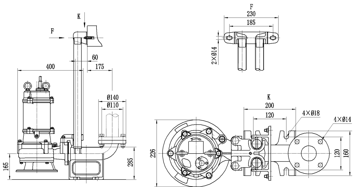
自动耦合式安装尺寸图
