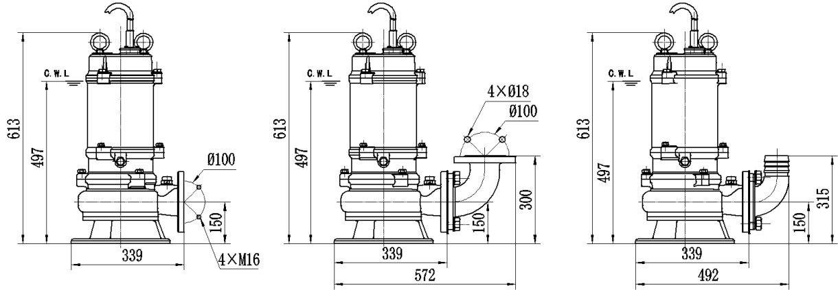
移动式安装尺寸图
